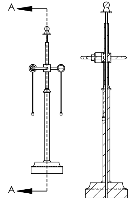
SECTION A-A SCALE 1 : 15
