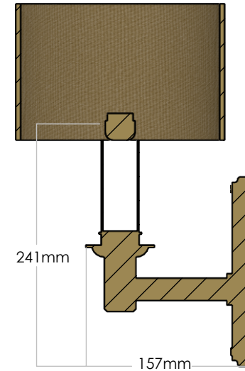
SECTION A-A SCALE 1 : 4
